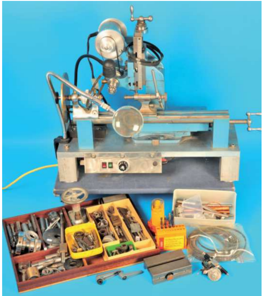
735 Massiver Eisentisch mit stabil aufgebauter Leinen WW Drehbank mit angebauter Fräsmaschine, große Teilscheibe mit 21 Teilkreisen, erhöhte Spitzenhöhe auf 60 mm, Wangenlänge 500 mm. Zahnriemenantrieb mit Bosch 12 Volt Gleichstrommotor, sehr massive Fräseinrichtung (5723) 1300,-
