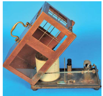
727 Thermograph auf Gussplatte mit Kup- ferdeckel und Traggriff, auf Werk sig- niert The Horstmann Gear Co. Ltd., in Bath, England, 7 Days, (7526), M = 27 x 13,5 x 16 cm ( ohne Traggriff) 240,-
