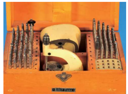
731 Boley-Triebnietmaschine in Holzkas- ten, mit nicht ganz komplettem Punzen- satz, ca. 100 Punzen (7215) 100,-
