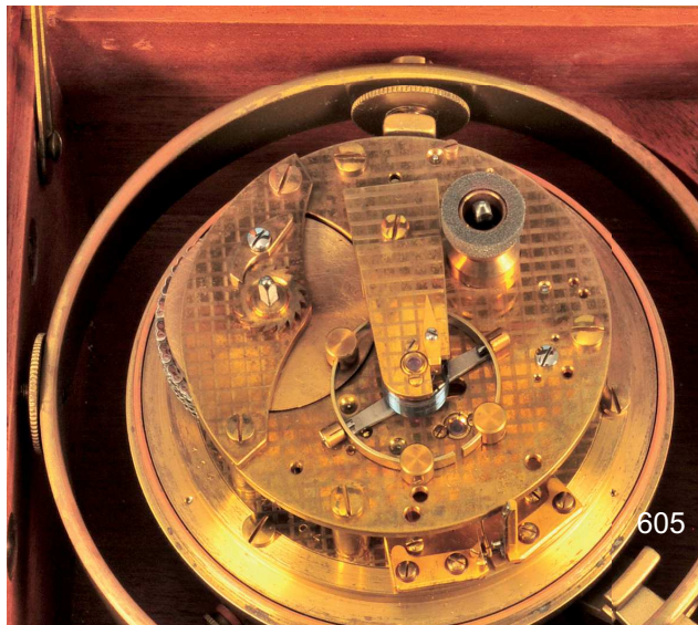
605 Marine-Chronometer, GUB, Glashütter Uhrenbetriebe, Kal. 100, Nr. 12104, im 2-tlg. Holzgehäuse mit seitlichen Traggriffen, kardanisch gelagertes Messinggehäuse, versilbertes Zifferblatt mit römischen Zahlen, kleine Sekunde bei der "6", Skala für 56-Std.-Gangreserve bei der "12", gebläute Zeiger, Werk mit Schnecke und Kette, Gegengesperr, Chronometerhemmung mit Feder, freischwingende, zylindrische Spirale, große Kompensationsunruh mit Ausgleichsgewichten, intakt (6441), M = 19 x 19 x 18,5 cm 1300,-
