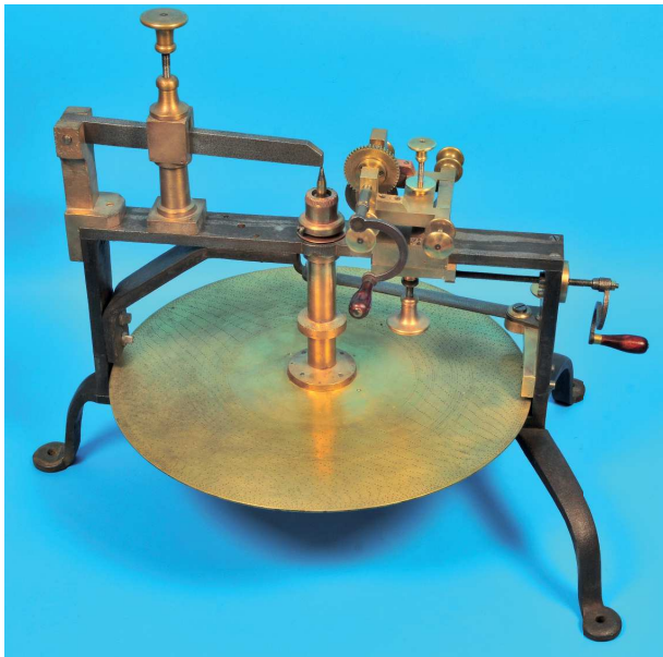
626 Große, antike Räderschneidmaschine , Eisen/Messing-Ausführung, große Teilscheibe, D = 50 cm, Kurbeln mit Holzgriffen (4915) 2200,-
