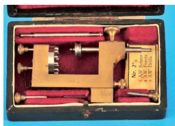
636 Feinbohrmaschinen im Original-Etui, bez. C.V.Z. (5867) 45,-
