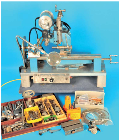
627 Massiver Eisentisch mit stabil aufgebauter Leinen WW Drehbank mit angebauter Fräsmaschine , große Teilscheibe mit 21 Teilkreisen, erhöhte Spitzenhöhe auf 60 mm, Wangenlänge 500 mm. Zahnriemenantrieb mit Bosch 12 Volt Gleichstrommotor, sehr massive Fräseinrichtung (5723) 1500,-
