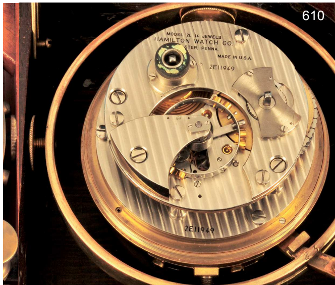
610 Hamilton-Marine-Chronometer, Modell 21 , im 3-tlg. Holzkasten mit Messing- ecken und Traggriffen, auf Gehäuseplakette, Werk und Zifferblatt sign. Hamilton, Lancaster U.S.A., Nr. ZE11949 , kardanisch gelagertes Messinggehäuse, versilbertes Zifferblatt mit arabischen Zahlen, kleine Sekunde, Skala für 56-Std. Gangreserve bei der "12", vernickeltes Werk mit Streifendekor und Transportsicherung, Modell 21, 14 Jewels mit Schnecke, Kette und Gegengesper, Chronometerhemmung mit Feder, sehr große Kompensationsunruh mit Ausgleichsschrauben, freischwingende, zylindrische Spirale, intakt, (6474), M = 19 x 19 x 19,5 cm 1500,-
