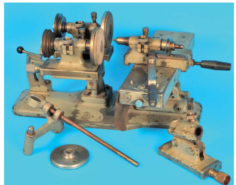
632 Alte, Maschine zur Anfertigung von Sonnenschliffen auf Kron- und Sperrädern . Zwei Spindeln und beweglicher Schlitten, Gebr. Sallas (5727) 250,-
