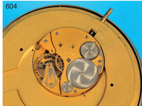
604 Flotten-Chronometer, Typ „B“, sign. A. Lange & Söhne, Glashütte b/Dresden, Nr. 206 326 B , vernickeltes Gehäuse im 2-tlg. Mahagoni-Holzkasten, versilbertes Zifferblatt mit arabischen Zahlen, kleine Sekunde bei der „6“, 56-Stunden-Gangreserve bei der „12“, vergoldetes Messingwerk, cal 48, mit Ankerhemmung, 16 Steine, Guillaume-Unruh mit Goldschrauben, Breguet-Spirale und Schwannenhals-Feinregulierung, Aufzugskrone bei der „4“, intakt(6437), D = 12,5 cm (Lunette), Holzkasten = 16,5 x 16,5 x 8 cm 1300,-
