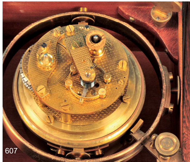
607 Deutsches Marine-Chronometer, signiert Hanseatische Werkstätten Friedrichs & Co., Hamburg-Schnelsen, Nr. 3011 (Lit. Abeler S. 192) 2-tlg. Holzgehäuse mit Holztraggriffen, kardanisch gelagertes Messinggehäuse, versilbertes Zifferblatt mit römischen Zahlen, kleine Sekunde bei der „6“, Skala für 56-Std.-Gangreserve bei der „12“, vergoldete Zeiger, vergoldetes Werk mit Schnecke, Kette und Gegengespierr, Chronometerhemmung mit Feder, Kompensationsunruh mit Ausgleichsgewichten, freischwingende, zylindrische Spirale, intakt (5296), M = 18,5 x 19 x 18 cm 1900,-
