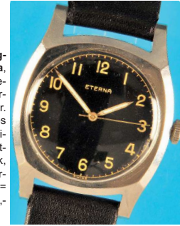
565 Militär Beobachtung-Armbanduhr, Eterna , gefertigt für die Tschechische Luftwaffe, verschraubtes Gehäuse Nr. 33577802, schwarzes Zifferblatt mit arabischen Zahlen, Leuchtzeiger, Ankerwerk, caliber 852S, 40er-Jahre intakt (6387) D = 39 mm 1200,-
