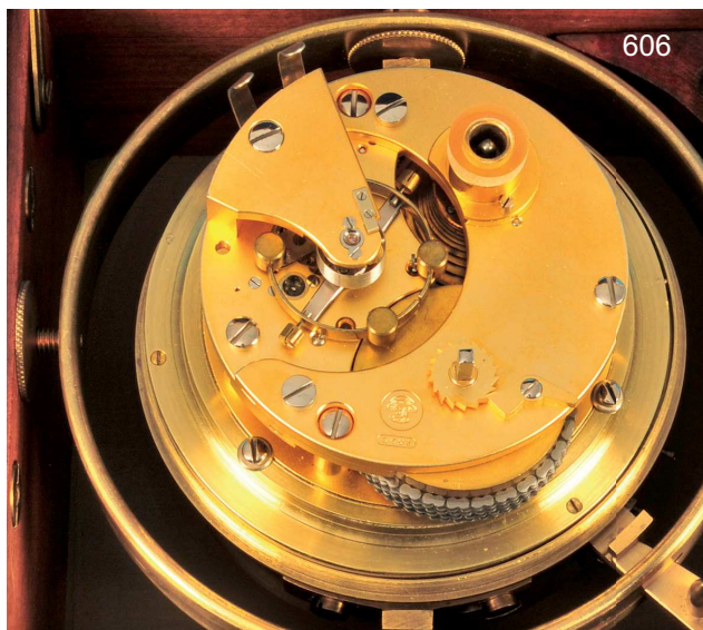
606 Marine-Chronometer Ulysse Nardin, Nr. 3601, auf Blatt sign. F.L.Löbner, Berlin.W., im 2-tlg. Holzgehäuse mit Traggriffen, kardanisch gelagertes Gehäuse, versilbertes Zifferblatt mit römischen Zahlen, kleine Sekunde, Skala für 56- Stunden-Gangreserve bei der "12", gebläute Zeiger, Werk mit Schnecke, Kette und Gegengesperr, Chronometerhemmung mit Feder, Kompensationsunruh mit Ausgleichsgewichten, freischwingende, zylindrische Spirale, Diamantdeckstein, intakt (6442), M = 18,5 x 18,5 x 18,5 cm 1800,-
